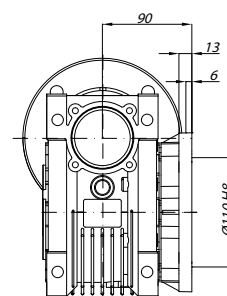
FB - FLANSZA DŁUGA
