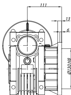
FA - FLANSZA KRÓTKA
