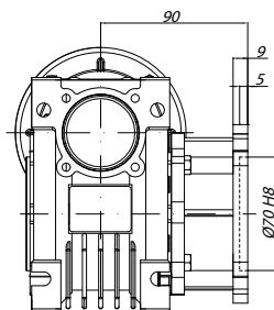
FA - FLANSZA KRÓTKA
