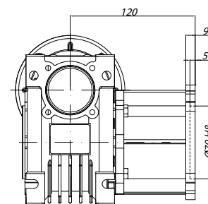
FB - FLANSZA DŁUGA
