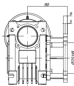
FA - FLANSZA KRÓTKA
